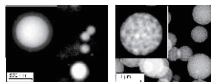
気相燃焼法で得られたコアシェルおよび不均質微粒子
