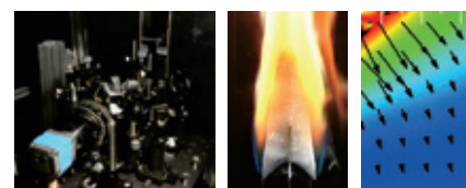
燃焼時の可燃性固体 (プラスチック) 内部非接触温度測定 (左: 測定装置, 中央: 燃焼時写真, 右: 内部温度分布)
