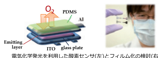
電気化学発光を利用した酸素センサ(左)とフィルム化の検討(右)
