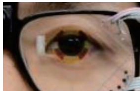
透過型の視線検出システム。極軽量・低消費電力での瞳孔位置計測が可能。
