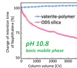
既存の充填剤との塩基性耐久性比較
