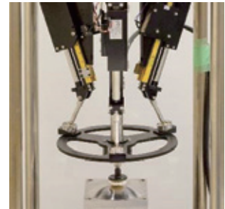
パラレルメカニズム研磨ロボット
