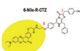
長波長発光用生物発光基質
