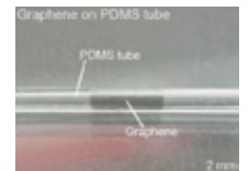
グラフェン素子による圧力センサ
