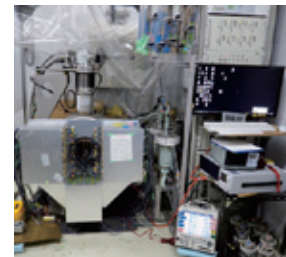
PEFCを計測するためのNMR計測装置
