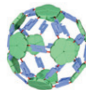
サッカーボール型タンパク質ナノ粒子TIP60のモデル構造
