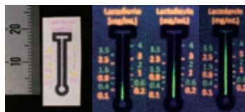
“温度計型”眼病マーカー検出用紙基板デバイス
