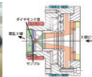
高温高圧セル 用途：X線回折、顕微鏡観察、FT-IR
