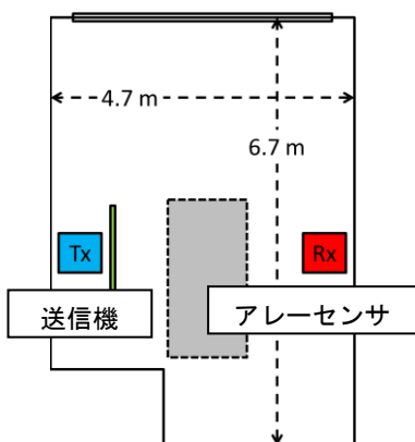
図 3 実験環境
